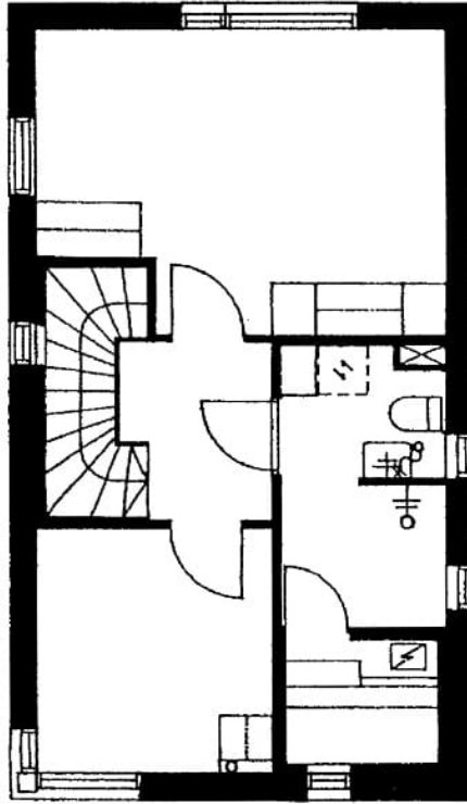
Verkkotie 1-5 D 14 / pohjakuva 2. kerros Not in scale
