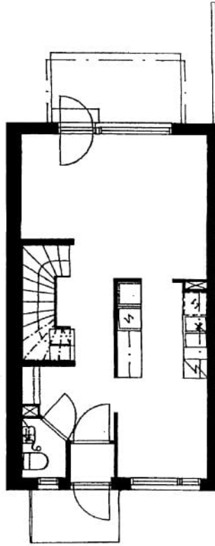
Verkkotie 1-5 D 14 / pohjakuva 1. kerros Not in scale
