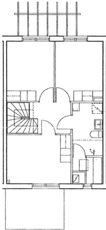
Rintalantie 7 D 22 / pohjakuva 2. kerros
