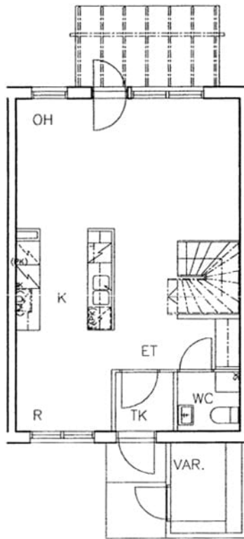
Rintalantie 7 C 14 / pohjakuva 1. kerros
