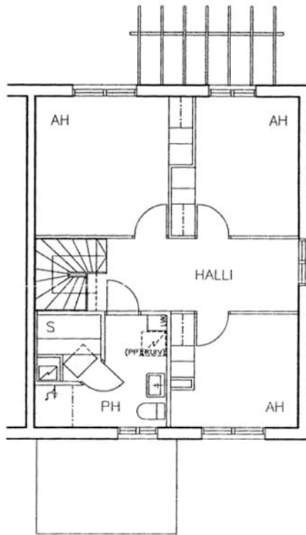
Rintalantie 7 C 13 / pohjakuva 2. kerros Ei mittakaavassa
