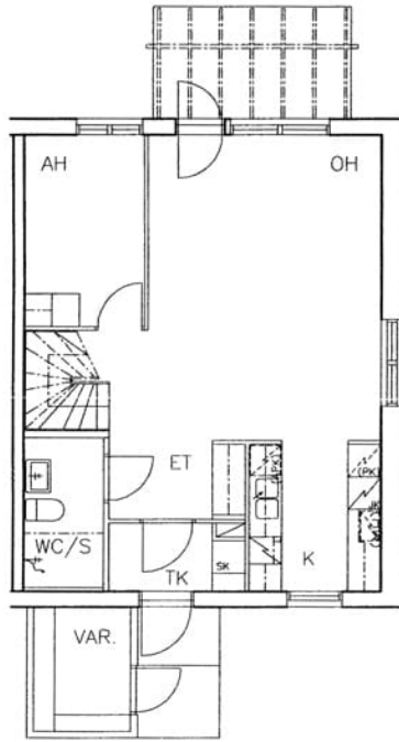
Rintalantie 7 A 6 / pohjakuva 1. kerros Ei mittakaavassa
