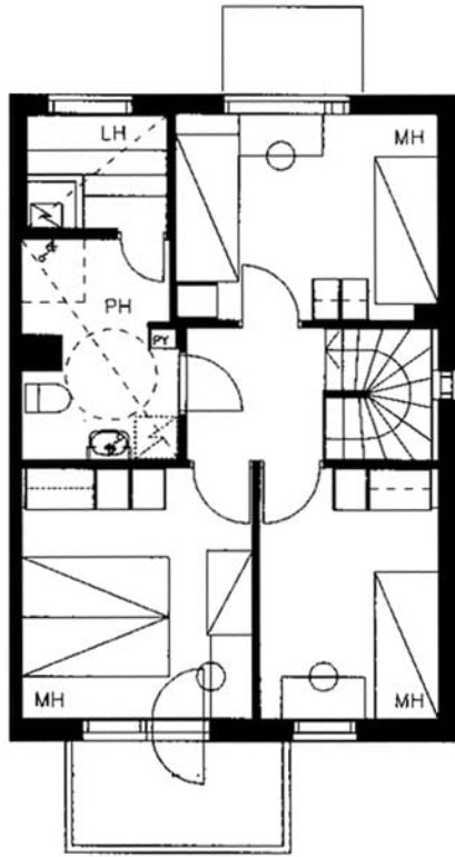
Luhtatie 6 C 12 / pohjakuva 2.kerros Ei mittakaavassa
