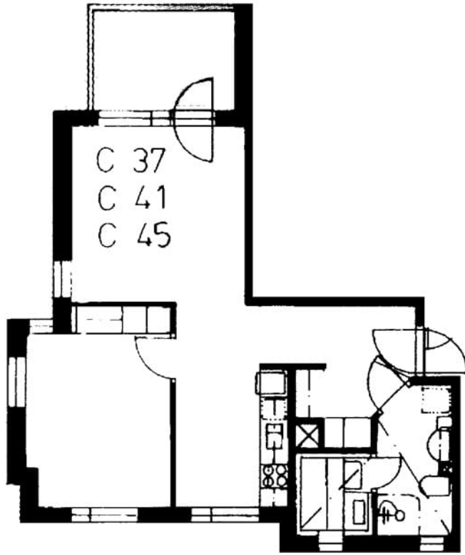
Pohjavedenkuja 3 C 45 / pohjakuva Not in scale
