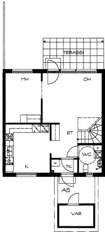
Pallotie 3 A 5 / pohjakuva 1. kerros Ei mittakaavassa
