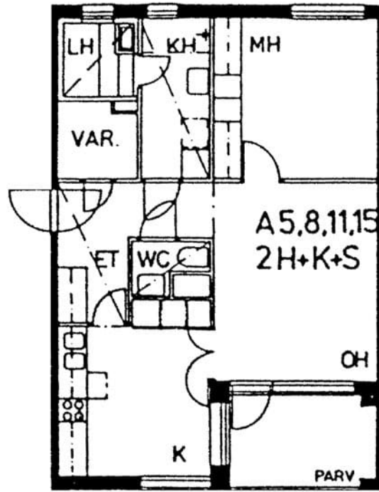
Linnanrakentajantie 11 A 11 / pohjakuva Ei mittakaavassa
