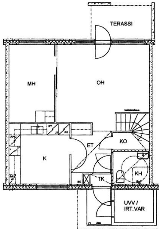
Ilotulitustie 12 H 25 / pohjakuva 1. kerros Ei mittakaavassa
