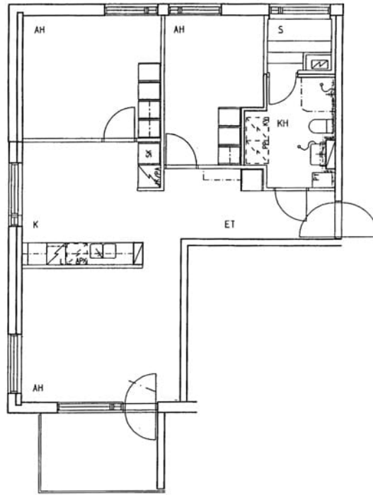
Lautamiehentie 2 A 25 / pohjakuva Not in scale
