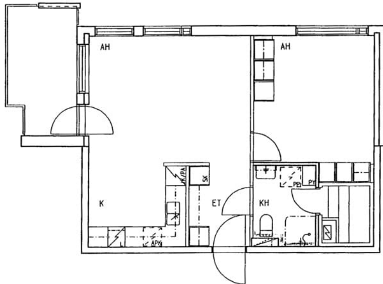
Lautamiehentie 2 A 14 / pohjakuva Ei mittakaavassa
