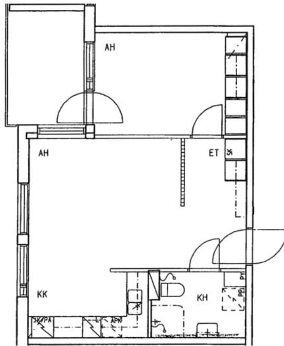
Lautamiehentie 2 B 56 / pohjakuva Ei mittakaavassa
