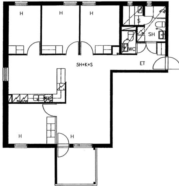
Joupintie 2 E 38 / pohjakuva Ei mittakaavassa
