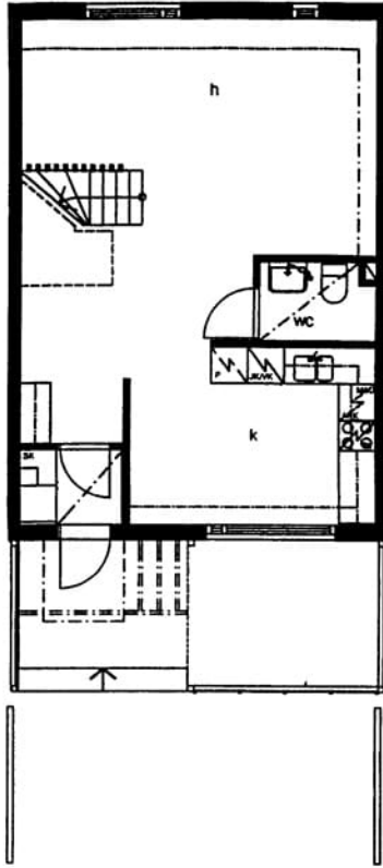
Norkkokuja 6 C 30 / pohjakuva 1. kerros Ei mittakaavassa
