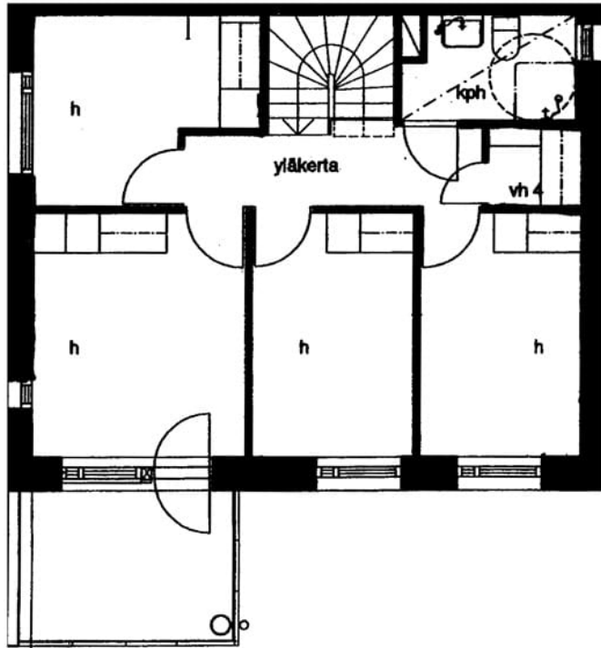
Norkkokuja 6 B 25 / pohjakuva 2. kerros Not in scale
