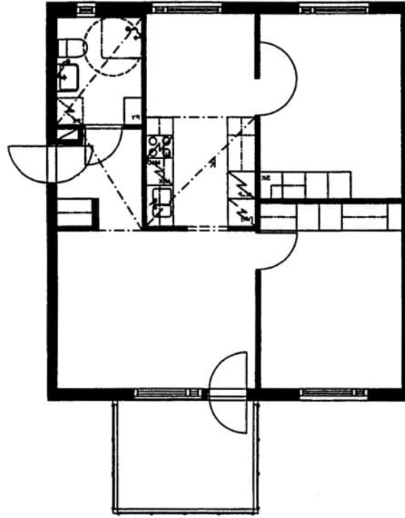
Norkkokuja 7 C 32 / pohjakuva Not in scale
