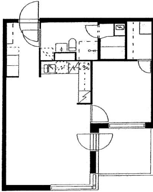
Vedenottamontie 12 E 45 / pohjakuva Not in scale
