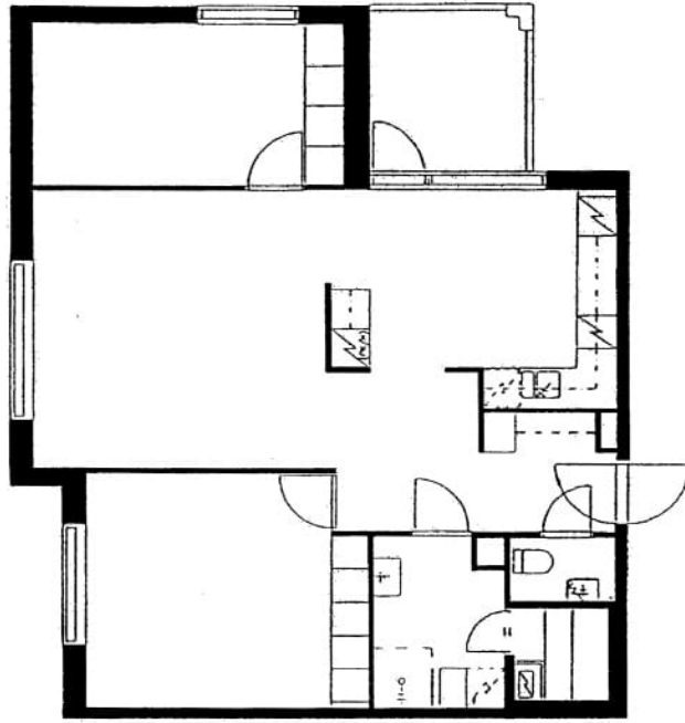
Vedenottamontie 12 D 26 / pohjakuva Not in scale
