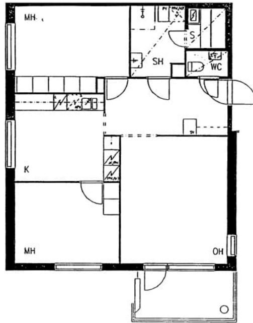
Vedenottamontie 12 D 28 / pohjakuva Not in scale
