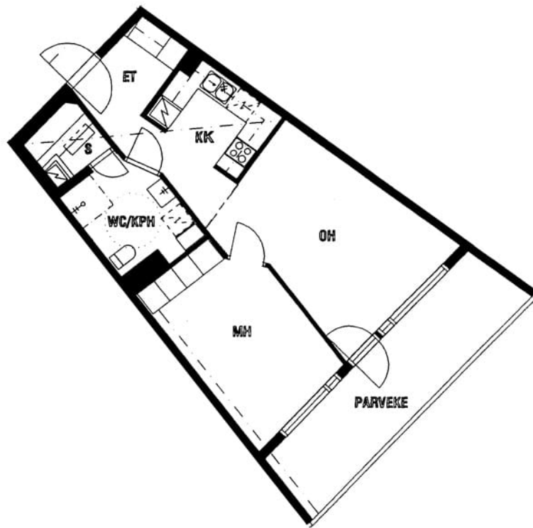
Paciuksenkaari 16 A 15 / pohjakuva Not in scale
