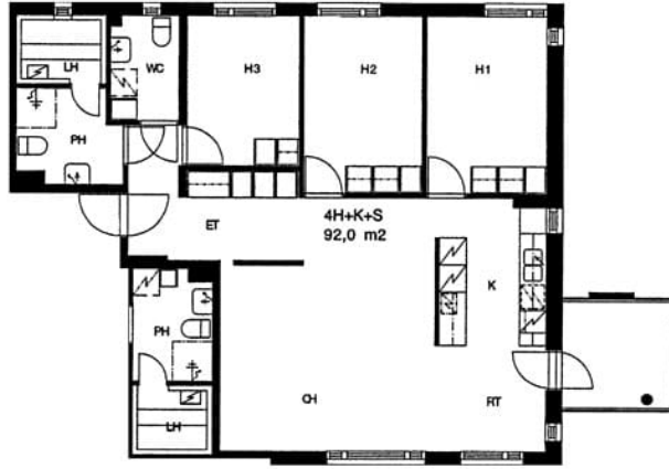
Lentokonetehtaankatu 12 A 18 / pohjakuva
