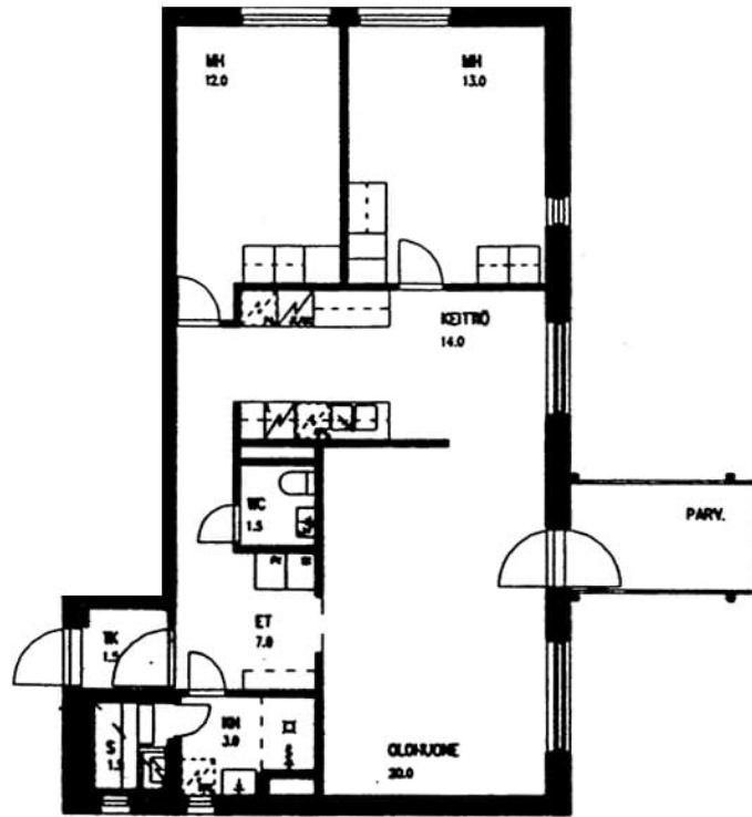
Taaplaajankatu 2 A 1 / pohjakuva Ei mittakaavassa
