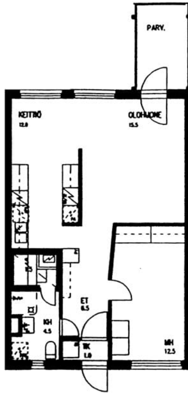
Taaplaajankatu 2 A 3 / pohjakuva Ei mittakaavassa
