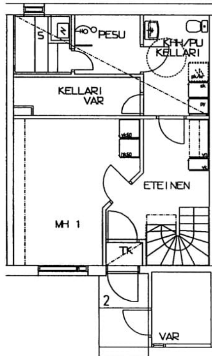
Pyytie 1 A 2 / pohjakuva 1. kerros Not in scale
