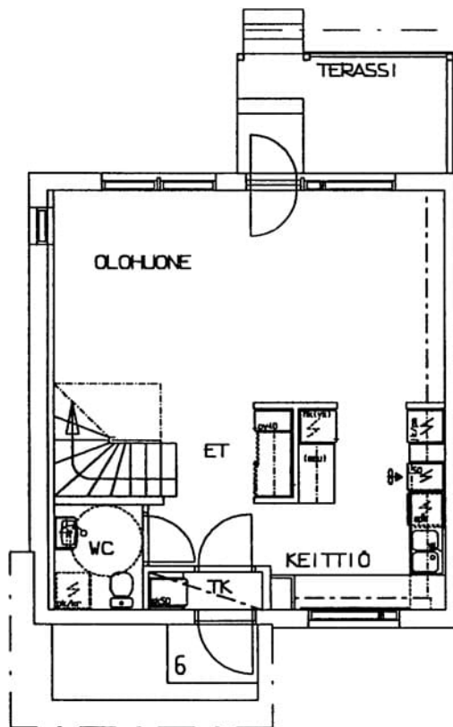
Pyytie 1 B 6 / pohjakuva 1. kerros Ei mittakaavassa
