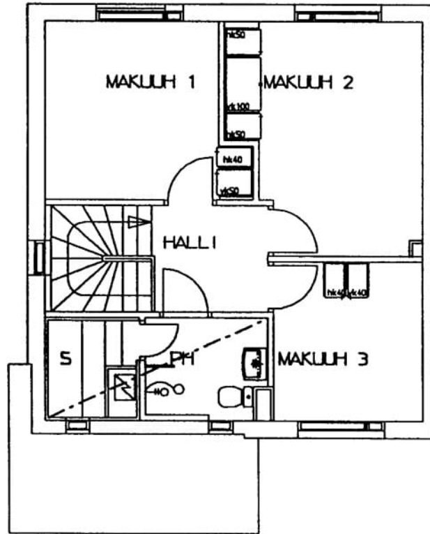
Pyytie 1 B 6 / pohjakuva 2. kerros Ei mittakaavassa
