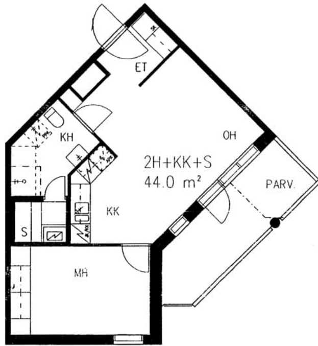
Palokorvenkatu 7 B 22 / pohjakuva Not in scale
