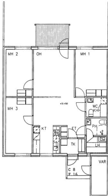
Kullerinkuja 1 C 8 / pohjakuva Ei mittakaavassa
