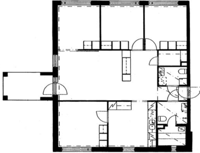
Takaniityntie 18 B 11 / pohjakuva Ei mittakaavassa
