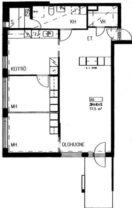
Takaniityntie 18 A 6 / pohjakuva
