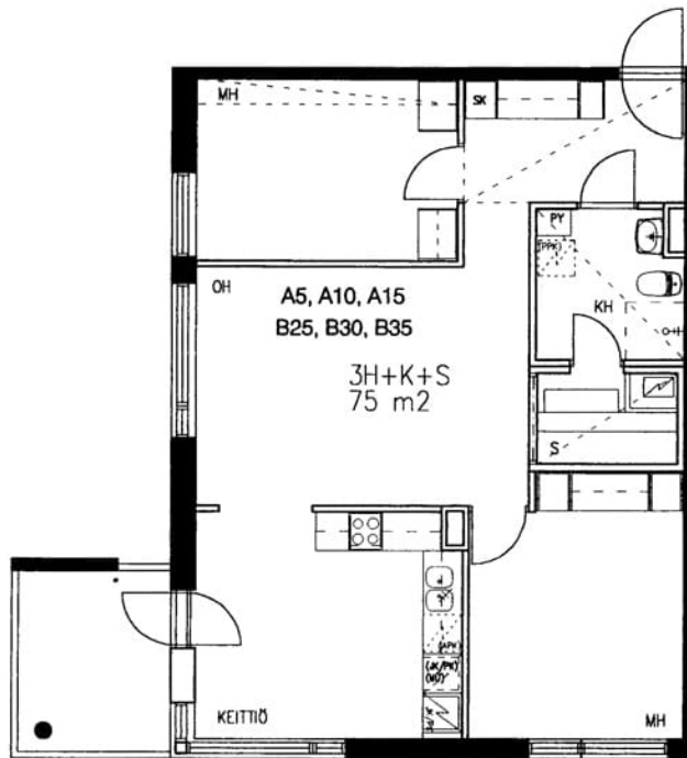
Ruusutorpantie 2 B 25 / pohjakuva
