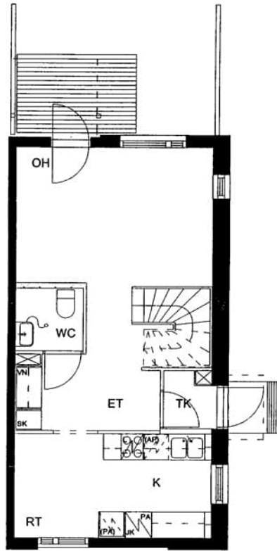
Fallbackantie 323 A 4 / pohjakuva 1.kerros Ei mittakaavassa
