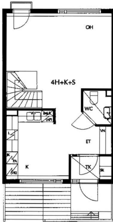
Nissaksentie 3 A 4 / pohjakuva 1. kerros Ei mittakaavassa
