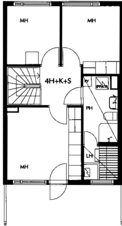
Nissaksentie 3 A 4 / pohjakuva 2. kerros Ei mittakaavassa
