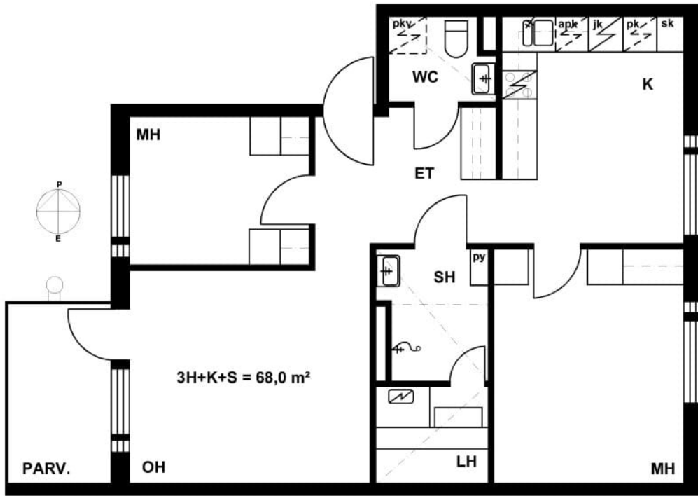
Piikuja 4 A 7 / Pohjakuva
