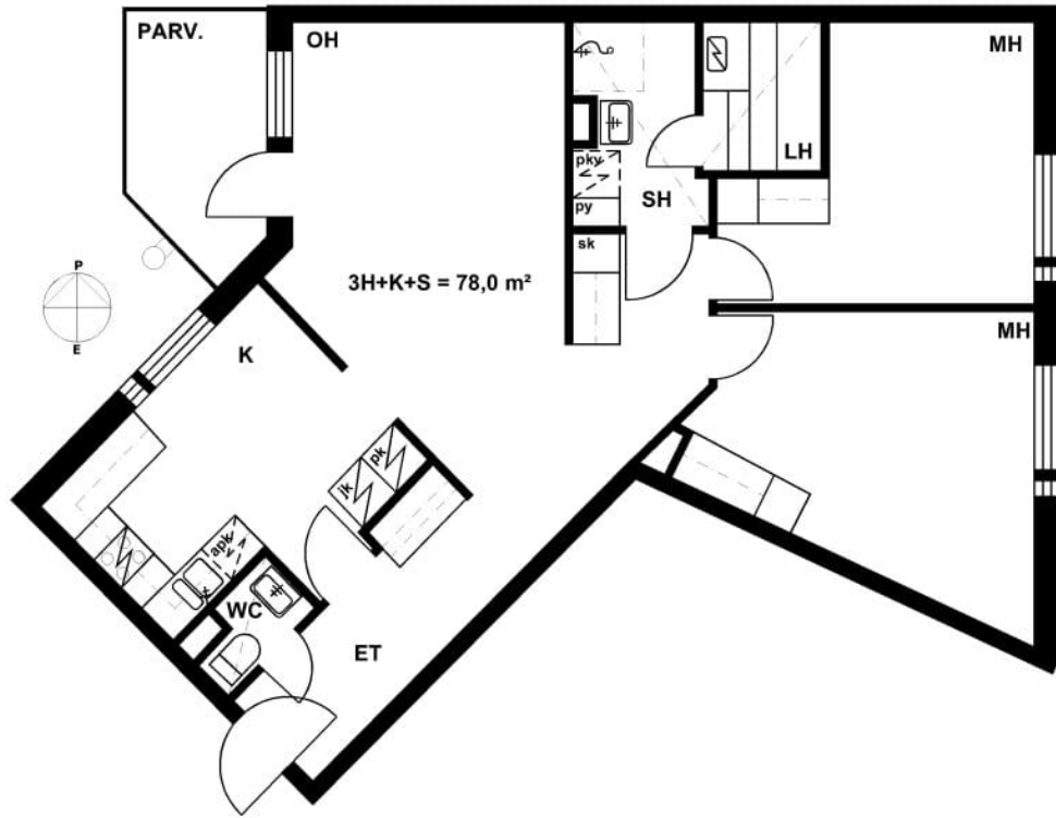
Piikuja 4 B 34 / Pohjakuva Ei mittakaavassa
