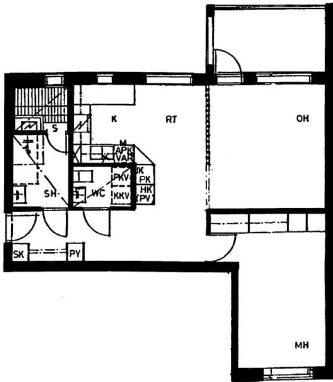
Haapakuja 3 B 25 / pohjakuva Not in scale
