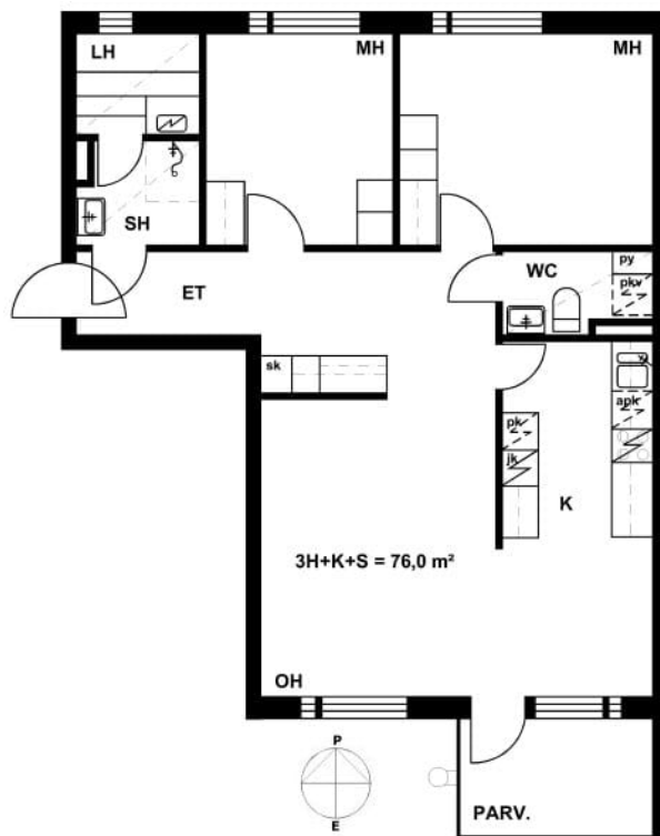
Piikuja 4 C 47 / Pohjakuva Ei mittakaavassa
