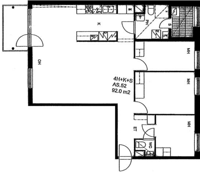
Vuosaarentie 1 C H 64 / pohjakuva Not in scale
