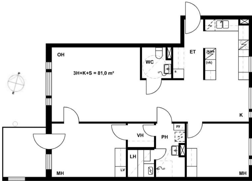
Itkonniemenkatu 3 B 23 / Pohjakuva Ei mittakaavassa
