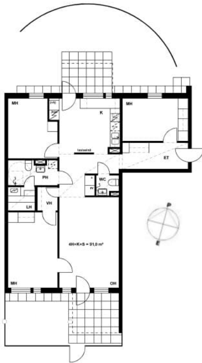
Itkonniemenkatu 3 C 47 / Pohjakuva Ei mittakaavassa
