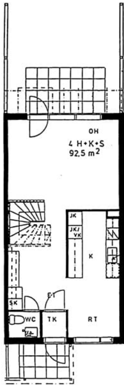
Kyläkaskentie 1 C 15 / pohjakuva 1. kerros Ei mittakaavassa
