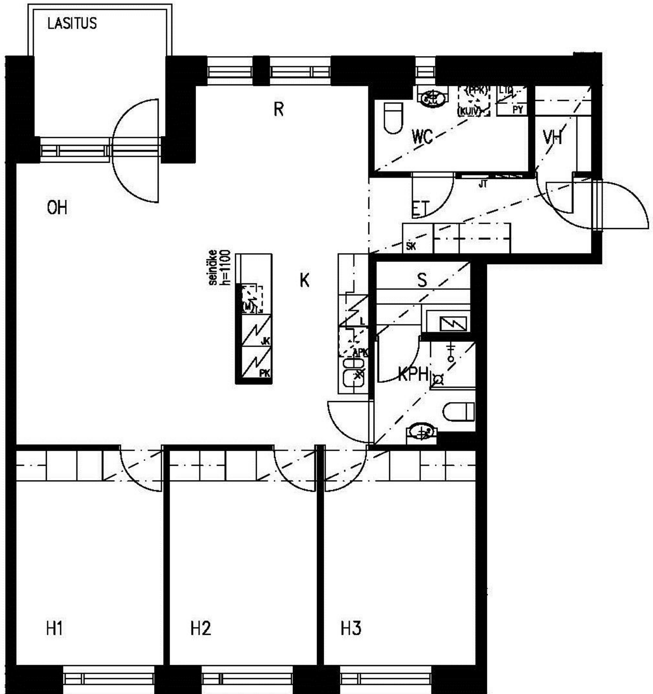
Purilaskuja 2 A 18 / Pohjakuva Ei mittakaavassa
