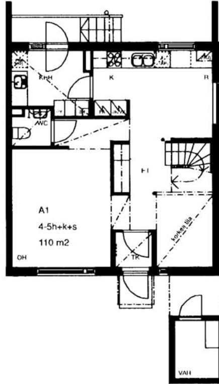
Pienenvillasaarentie 13 B 7 / pohjakuva 1. kerros Not in scale
