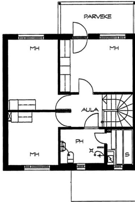
Jakomäentie 9 A 5 / pohjakuva 2. kerros
