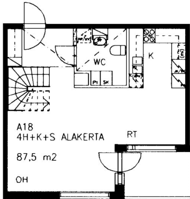
Nelikkotie 14 A 18 / pohjakuva 1.kerros Ei mittakaavassa
