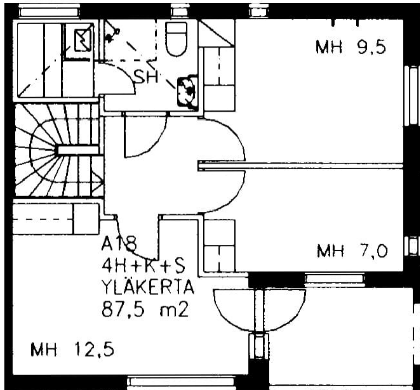
Nelikkotie 14 A 18 / pohjakuva 2.kerros
