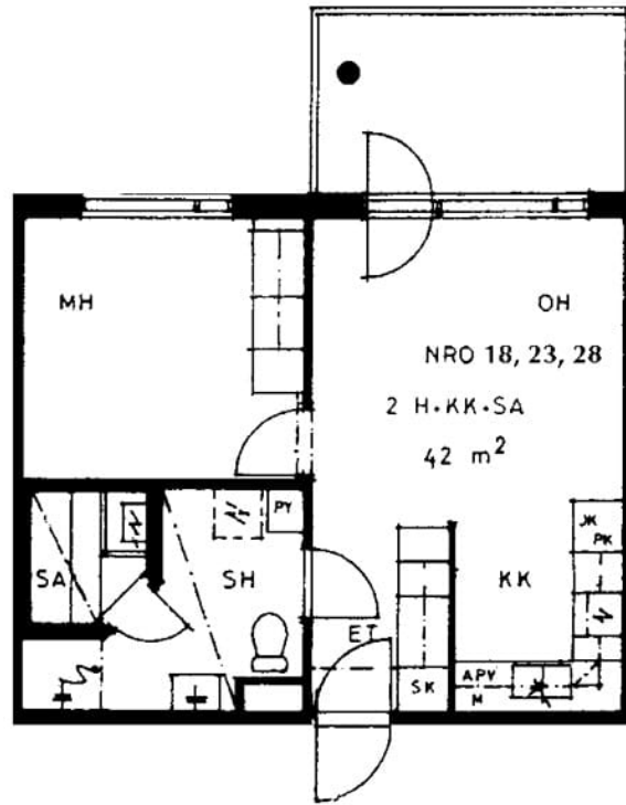
Peijaksentie 27 B 28 / pohjakuva Not in scale
