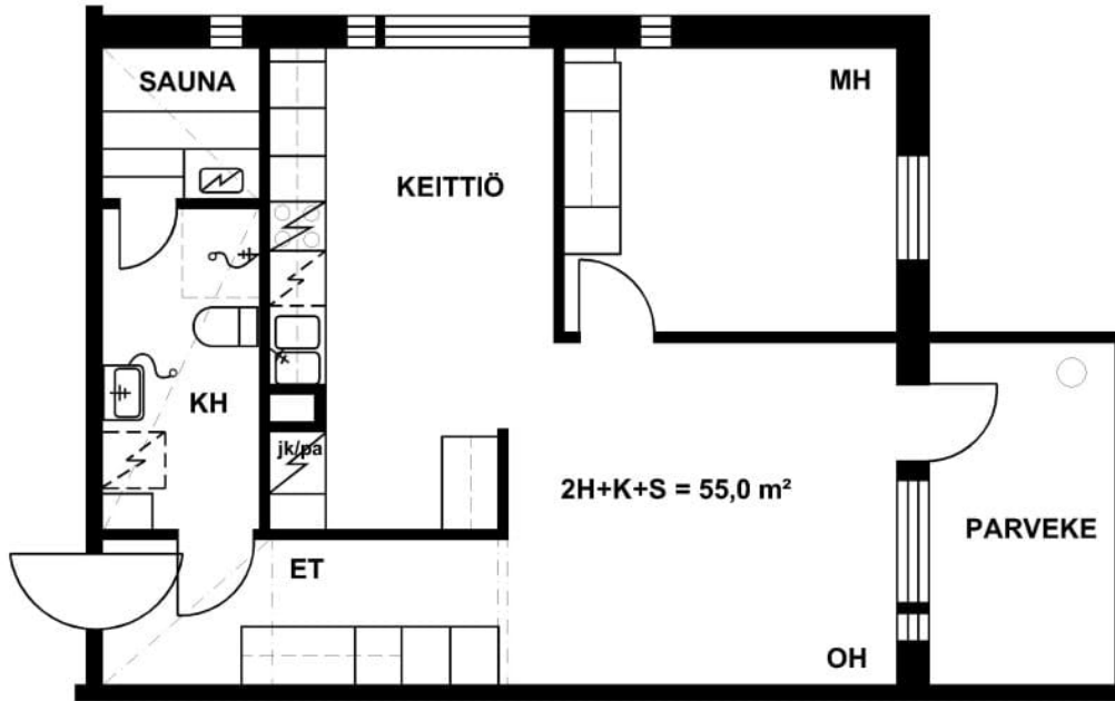
Maikkulanraitti 2 A 5 / Pohjakuva
