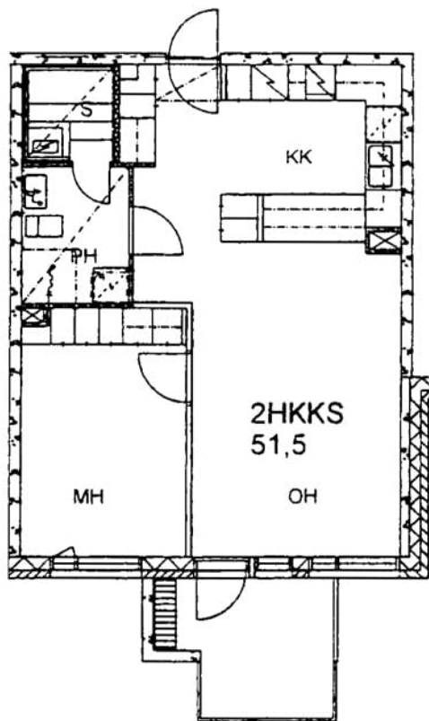
Kangaskontiontie 1 A 13 / pohjakuva Ei mittakaavassa
