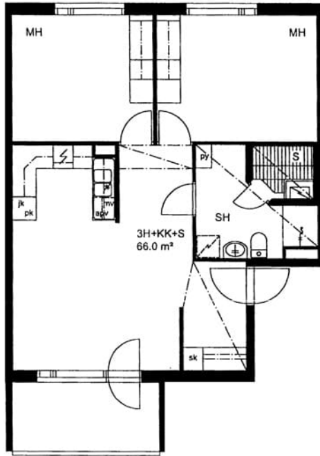
Vasamakatu 5-7 B 26 / pohjakuva Ei mittakaavassa
